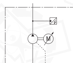
Single Displacement Type ASE *
